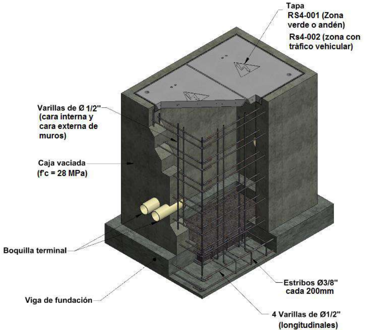
Esquema 6: Cajas vaciadas en concreto – Refuerzo en los muros
