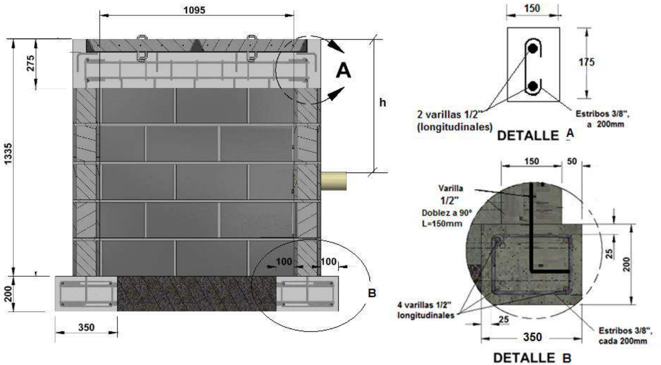
Esquema 11: Cajas en bloque de concreto – Sección transversal y detalle
