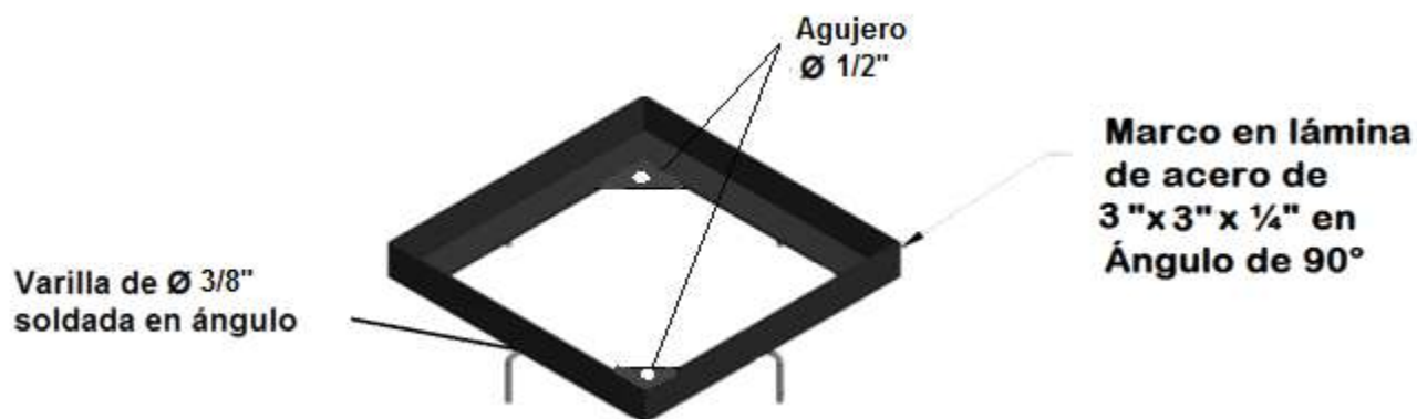
Esquema 13: Marco en lámina de acero –Vista en planta
