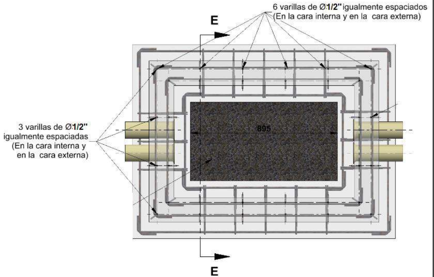
Esquema 7: Cajas vaciadas en concreto – Refuerzo en los muros
