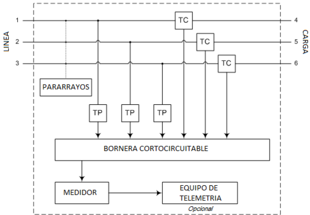
Figura 20. Principio de funcionamiento del sistema combinado
