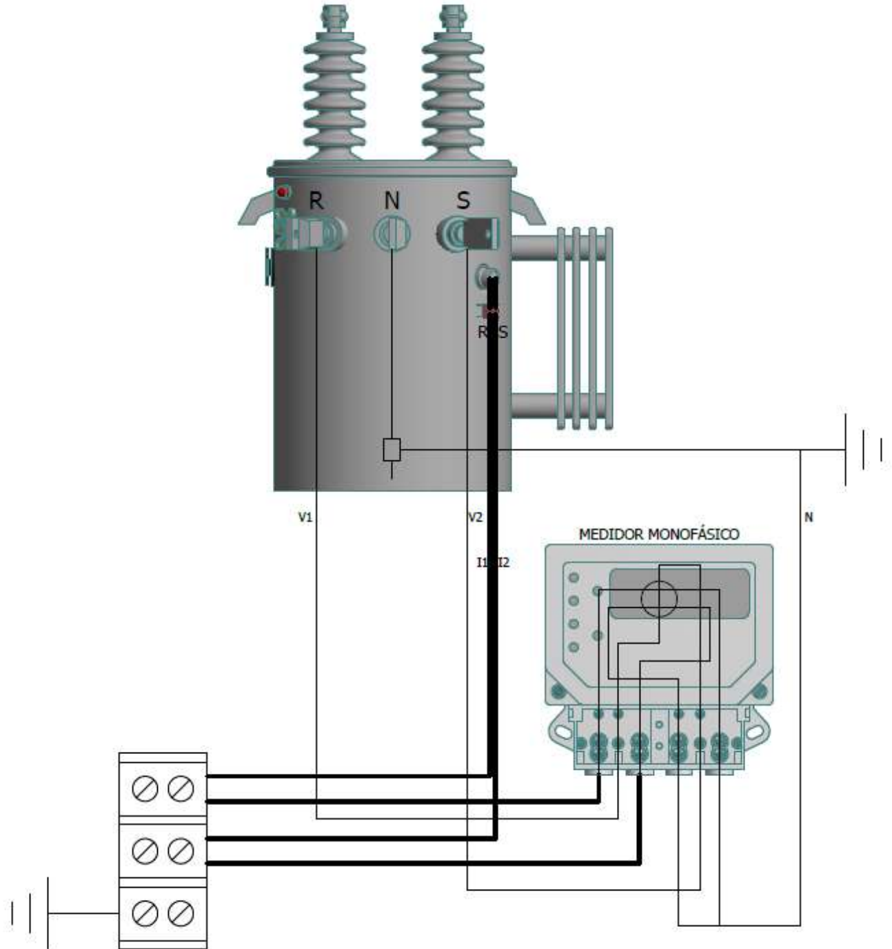
Figura 6. Diagrama de conexión Macromedición con medida semi-directa en transformador monofásico medidor de conexión simétrica o americana. Transformadores nuevos con TCs internos.
