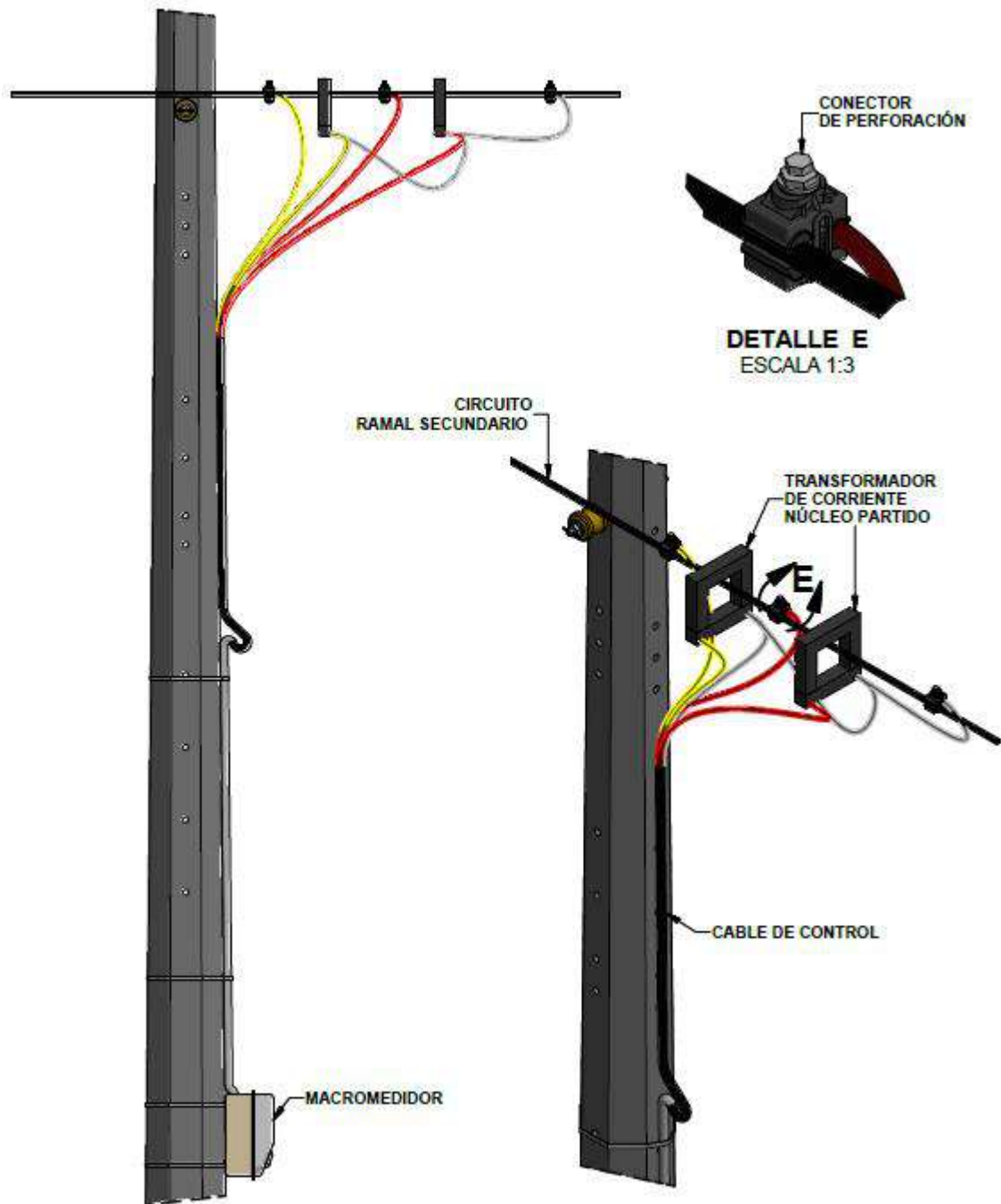
Figura 18. Instalación de macromedición en un circuito ramal
