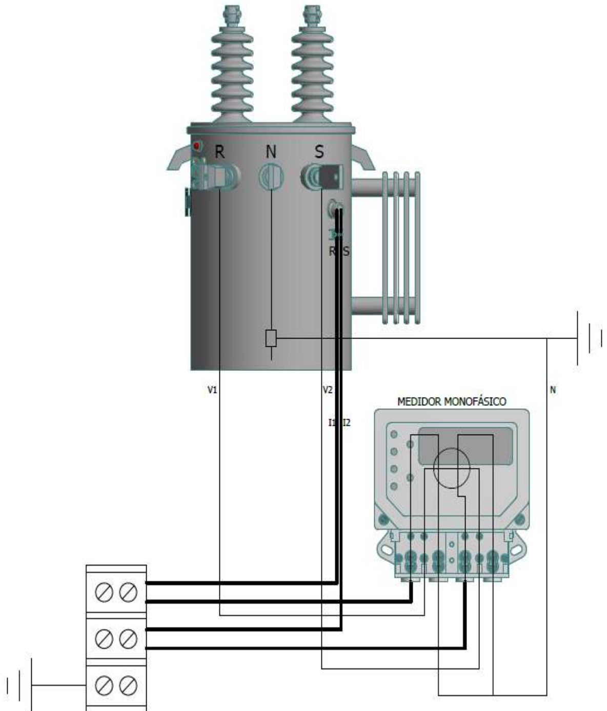
Figura 4. Diagrama de conexión Macromedición con medida semi-directa en transformador monofásico medidor de conexión asimétrica o europea. Transformadores nuevos con TCs internos.
