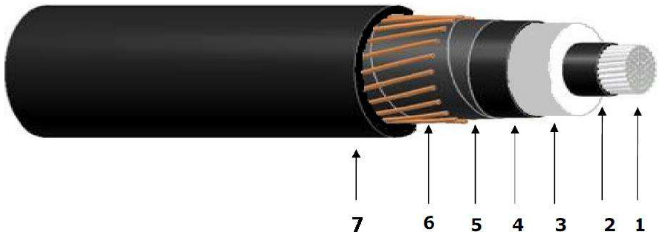
Figura No. 1 – Conformación cable de media tensión
